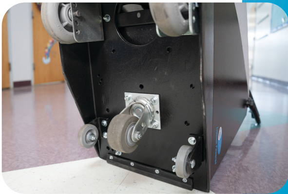
Roue arrière pivotante pour une manœuvrabilité accrue
